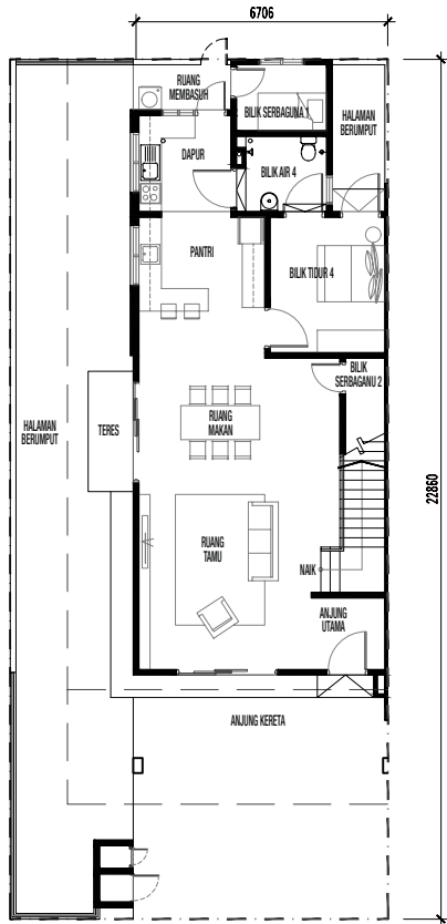
TINGKAT BAWAH
