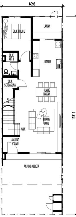
TINGKAT BAWAH
