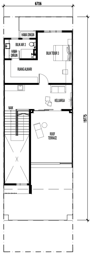
TINGKAT DUA
