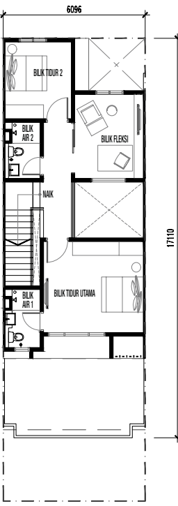
TINGKAT ATAS
