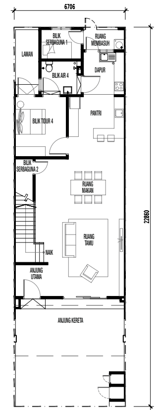
TINGKAT BAWAH
