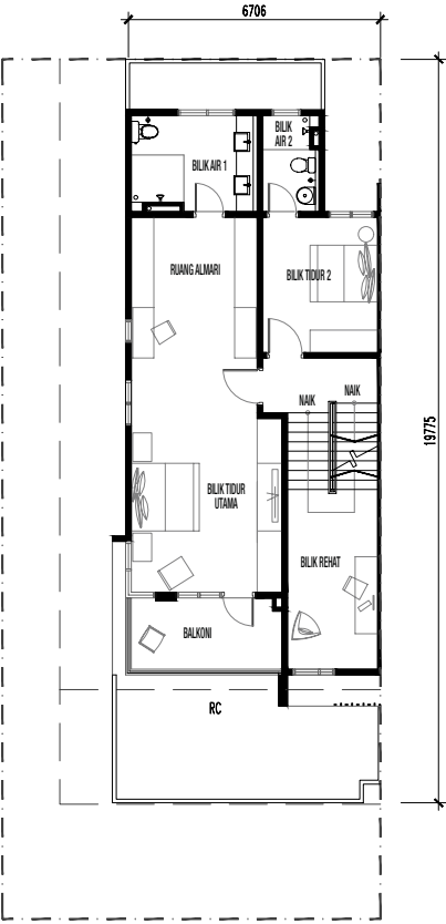
TINGKAT SATU
