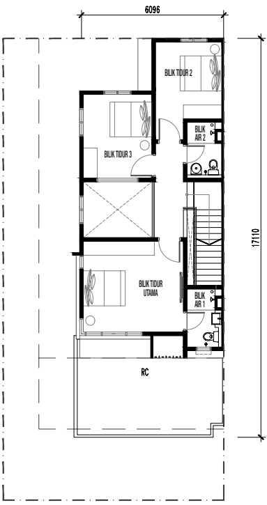
TINGKAT ATAS
