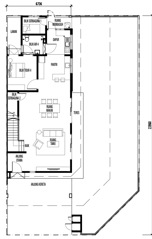
TINGKAT BAWAH
