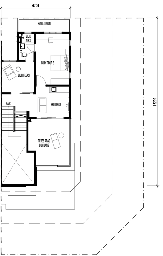
TINGKAT DUA
