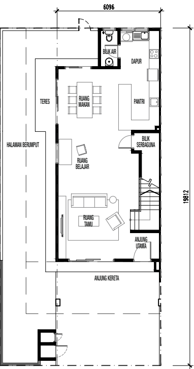
TINGKAT BAWAH
