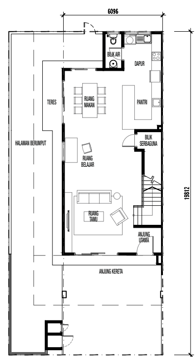
TINGKAT BAWAH
