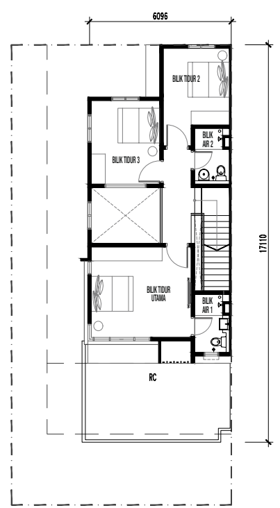
TINGKAT ATAS
