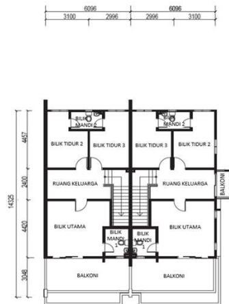
Pelan Lantai Tingkat Atas
