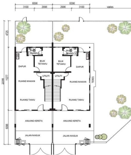
Pelan Lantai Tingkat Bawah
