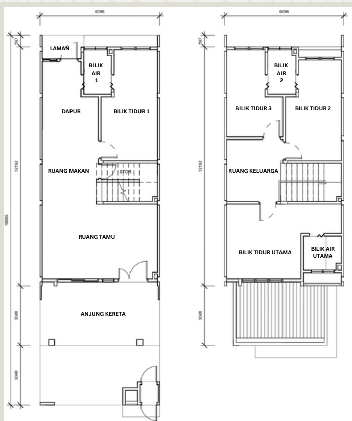
RUMAH TERES 2 TINGKAT
