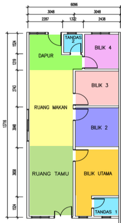
RUMAH TERES SETINGKAT Keluasan Lantai: 900 kaki persegi / 20' x 45'
