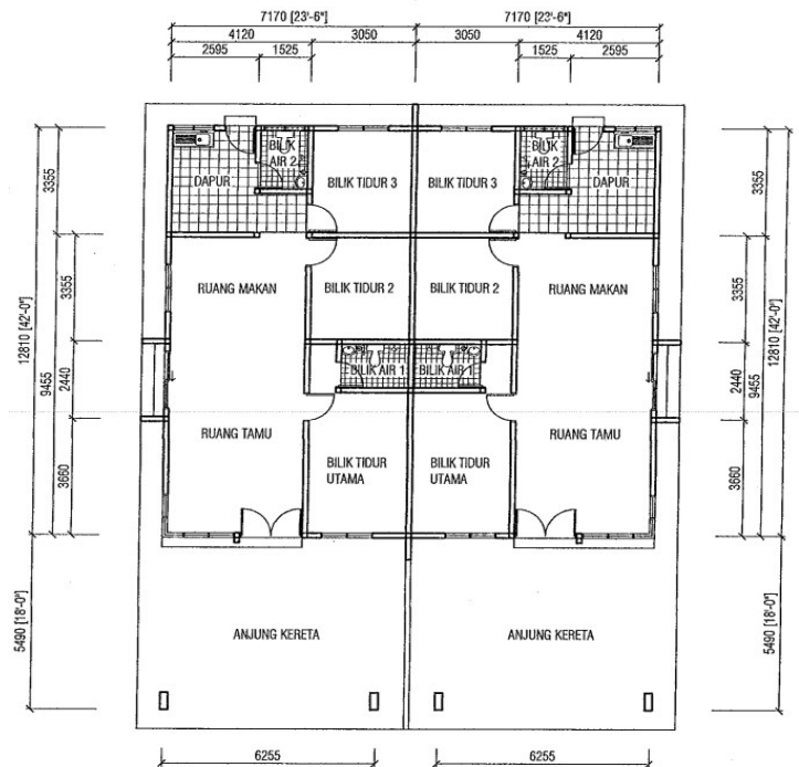
PELAN LANTAI
