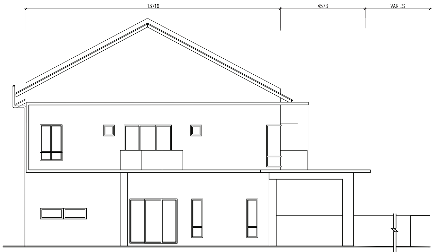
PANDANGAN SISI
