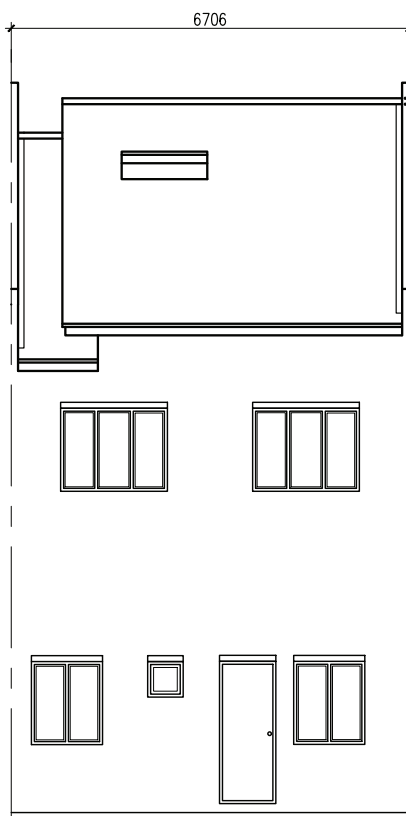
PANDANGAN BELAKANG
