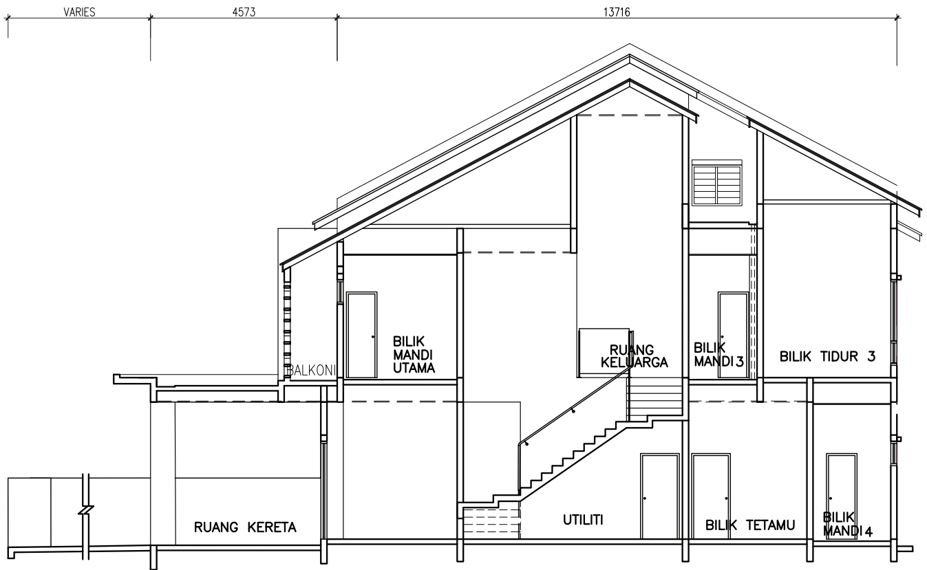
KERATAN
