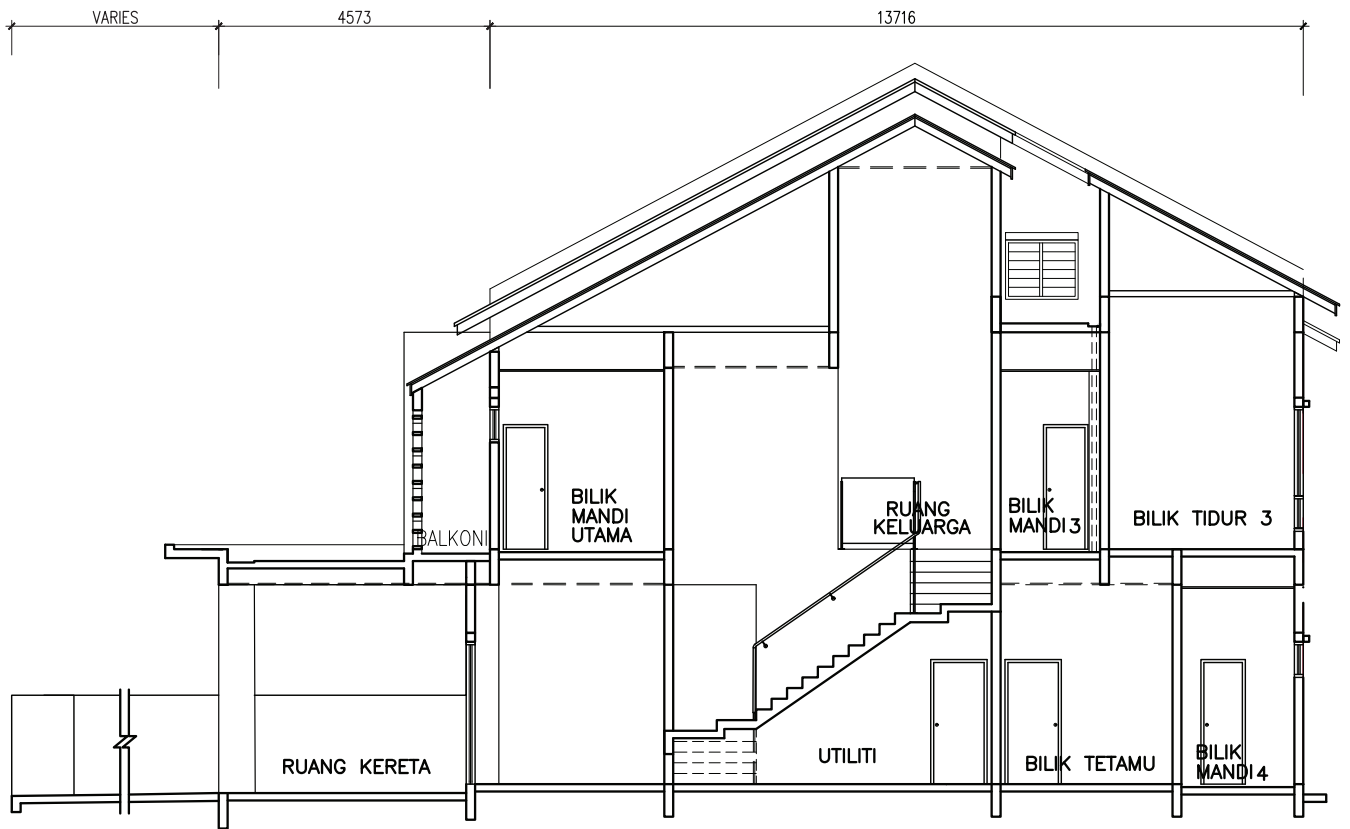
KERATAN
