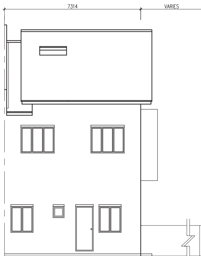
PANDANGAN BELAKANG
