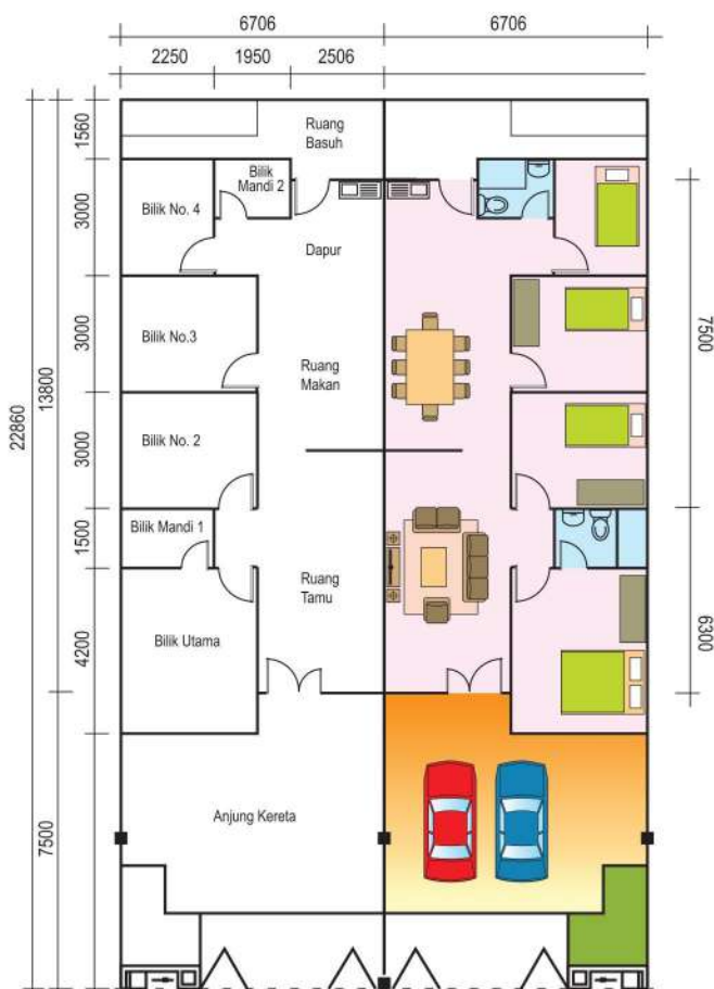
Pelan Lantai
