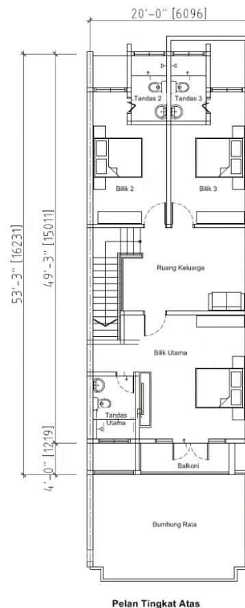
Pelan Tingkat Atas
