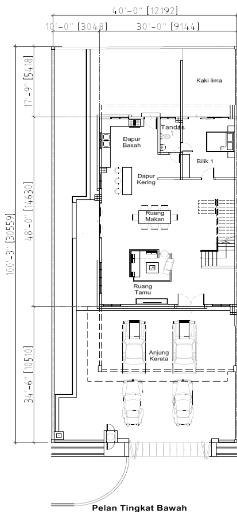
Pelan Tingkat Bawah
