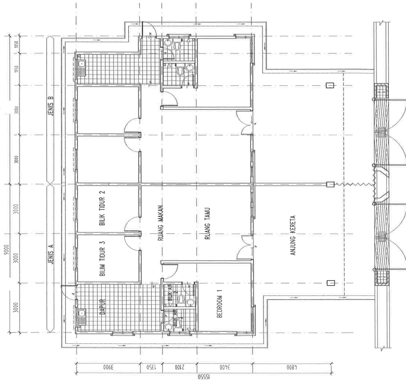
PELAN LANTAI
