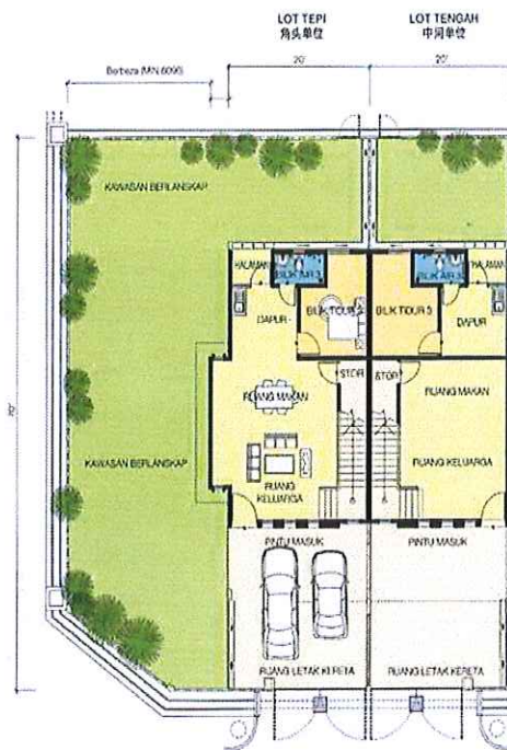
TINGKAT BAWAH 楼下平面图
