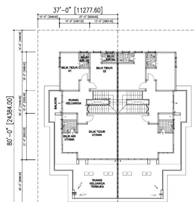
PELAN TINGKAT SATU | JENIS - A 37' X 80'
