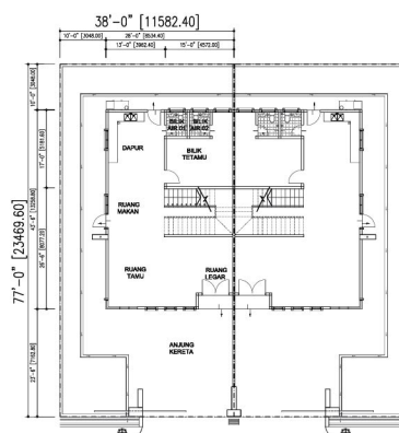
PELAN TINGKAT BAWAH | JENIS - B 38' X 77'
