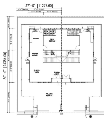
PELAN TINGKAT BAWAH | JENIS - A 37' X 80'
