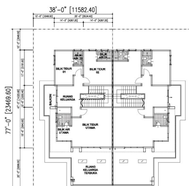
PELAN TINGKAT SATU | JENIS - B 38' X 77'
