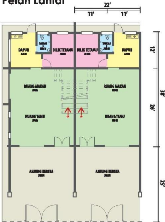
PELAN LANTAI BAWAH
