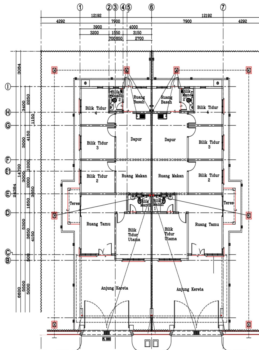
RUMAH BERKEMBAR 1 TINGKAT (40' X 80')
