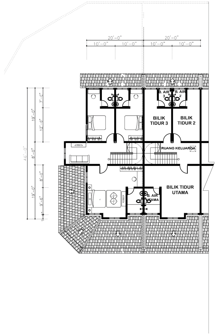
Tingkat Atas
