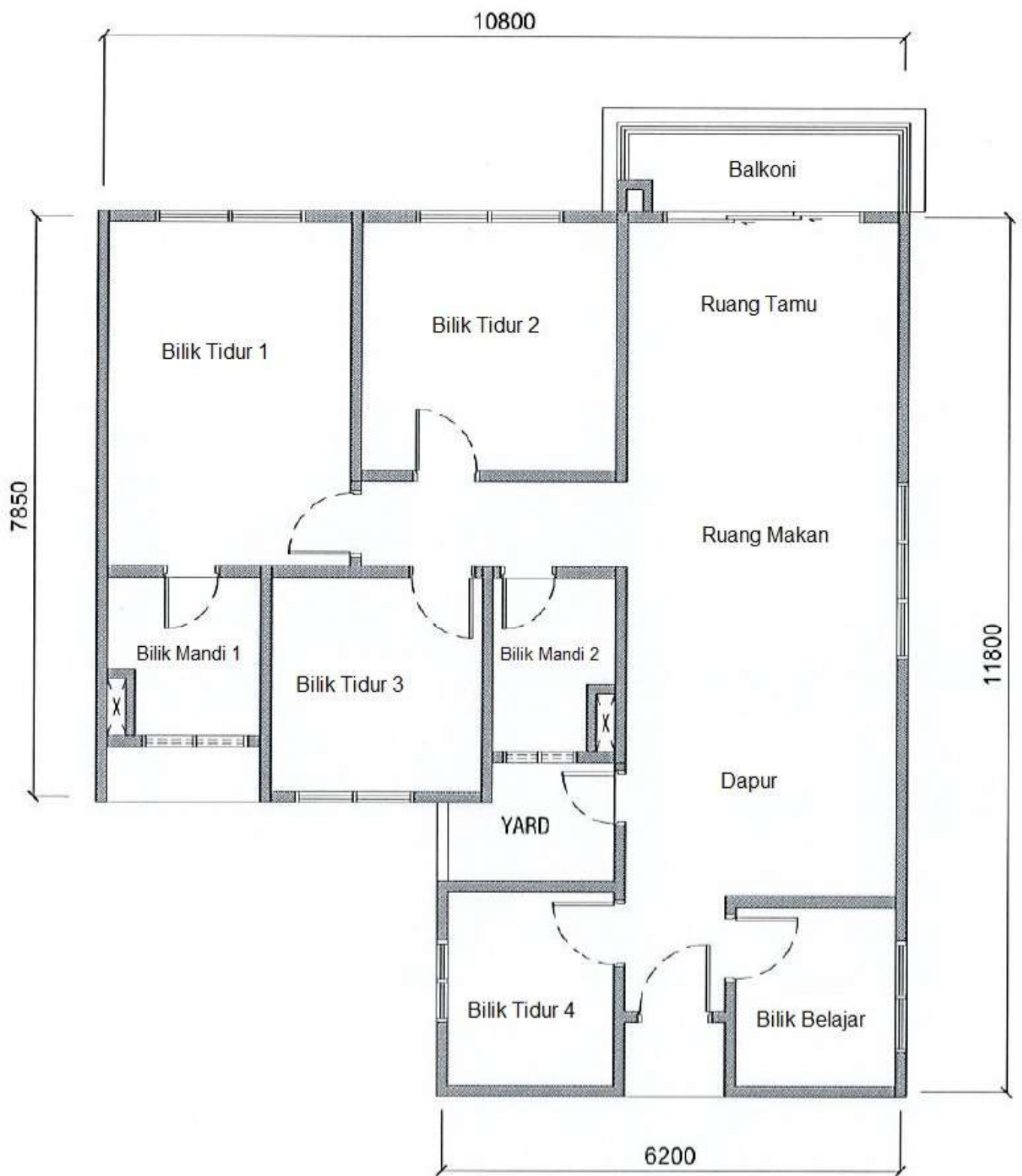
PELAN TIPIKAL JENIS C (MIRROR)
