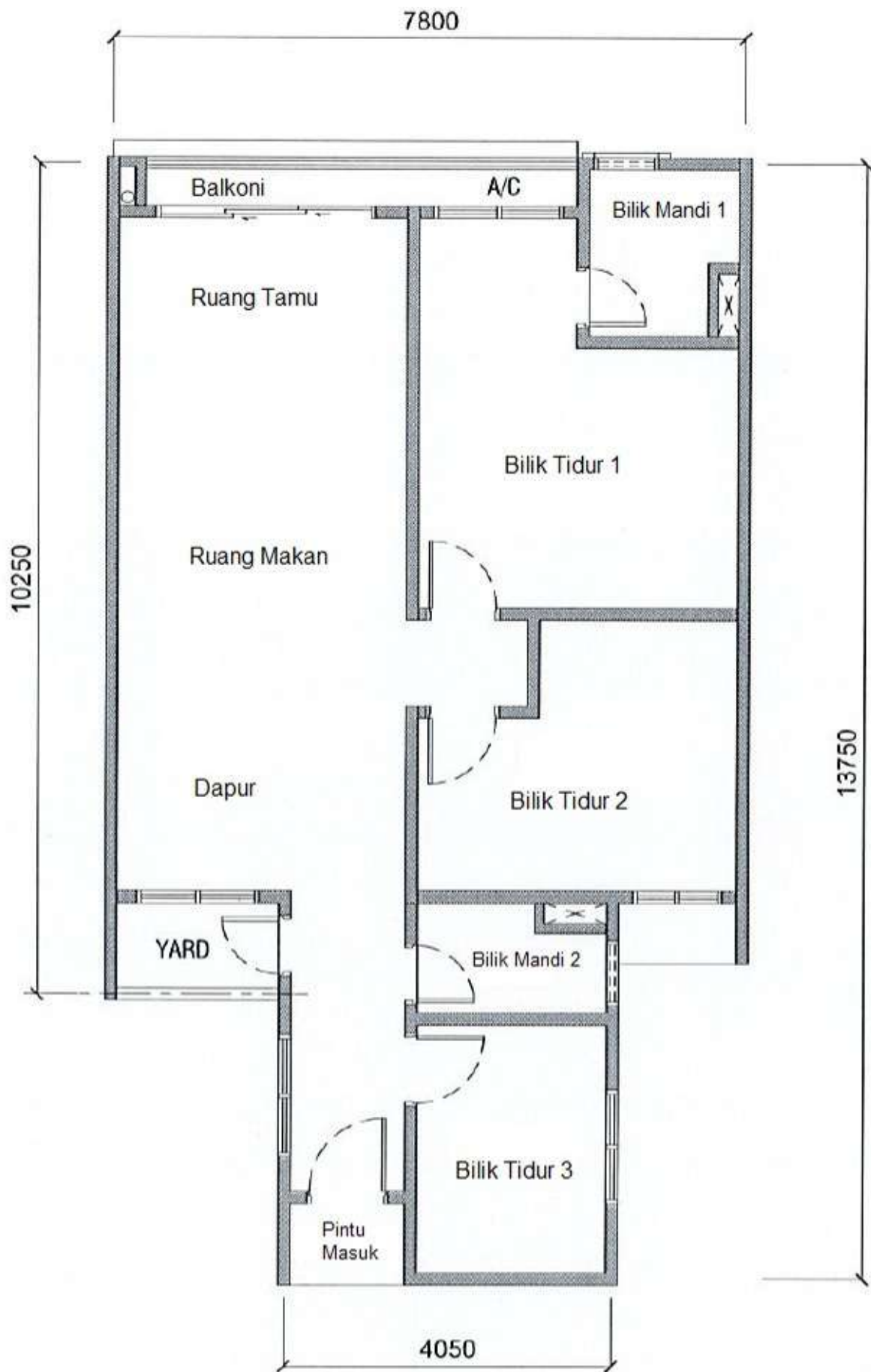
PELAN TIPIKAL JENIS A (MIRROR)
