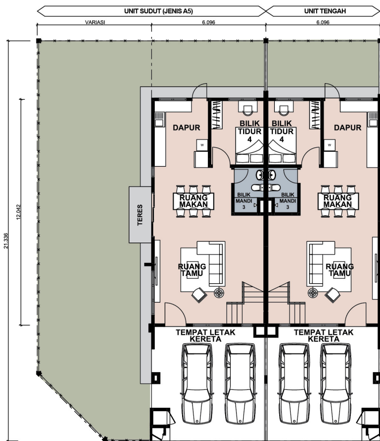
TINGKAT BAWAH
