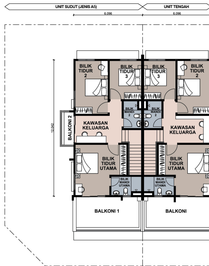
TINGKAT SATU
