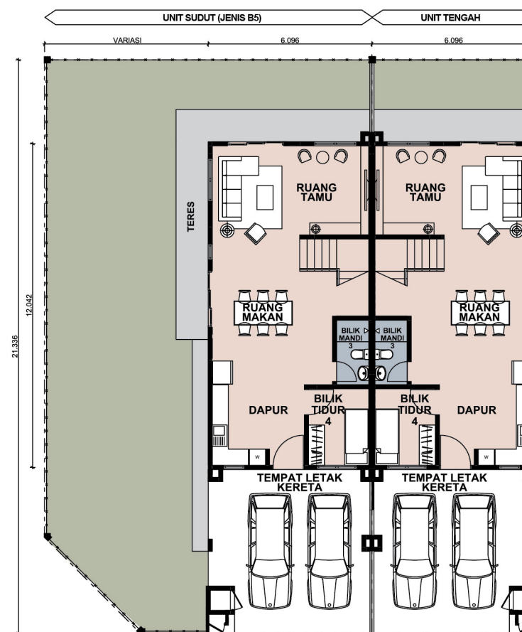
TINGKAT BAWAH
