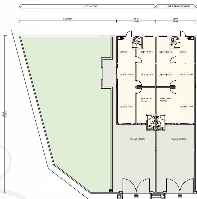
RUMAH TERES 1 TINGKAT (JENIS B) - 20' X 80'
