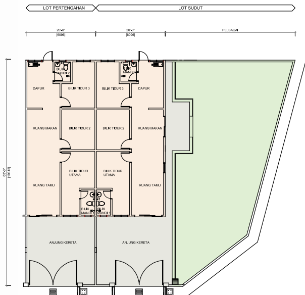
RUMAH TERES 1 TINGKAT (JENIS A) - 20' X 65'
