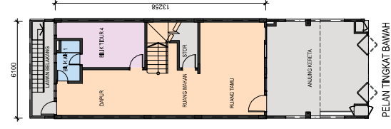
PELAN TINGKAT BAWAH
