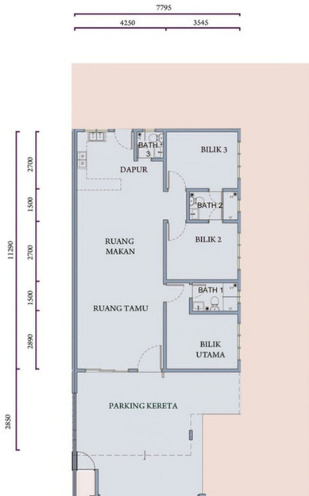
Pelan Lantai
