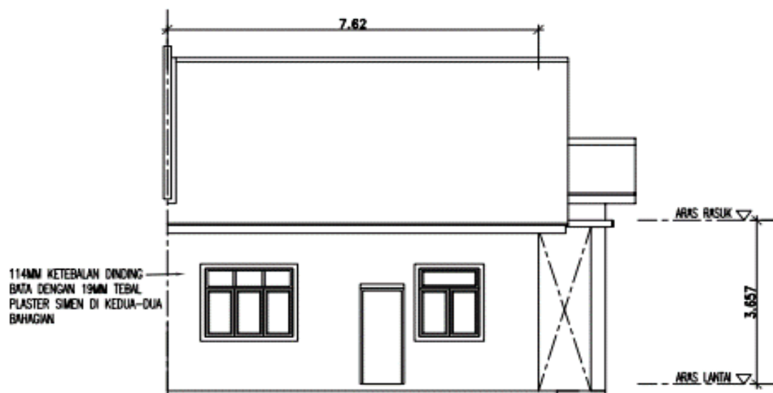
PANDANGAN BELAKANG
