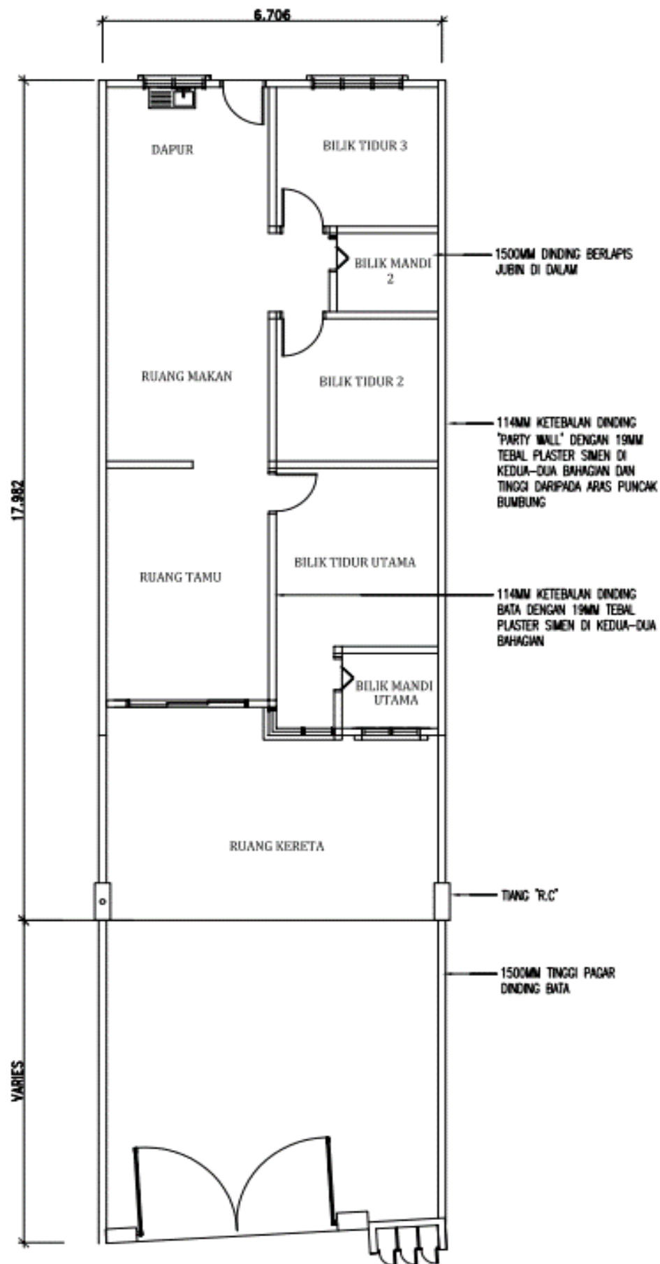
PELAN LANTAI Rumah Teres 1 Tingkat
