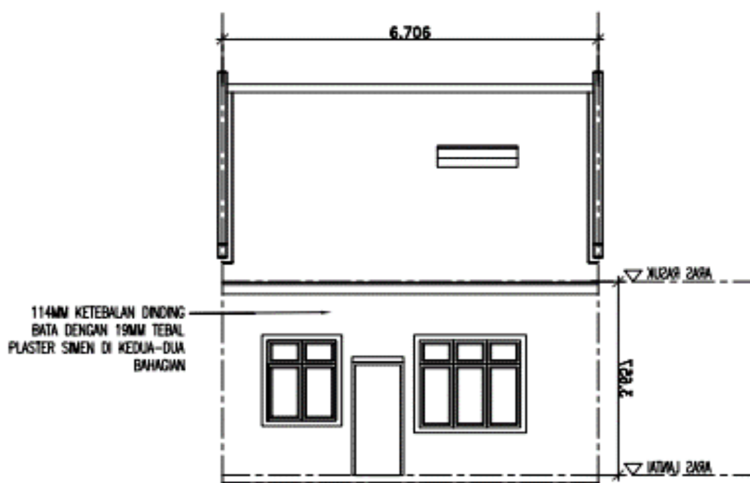
PANDANGAN BELAKANG
