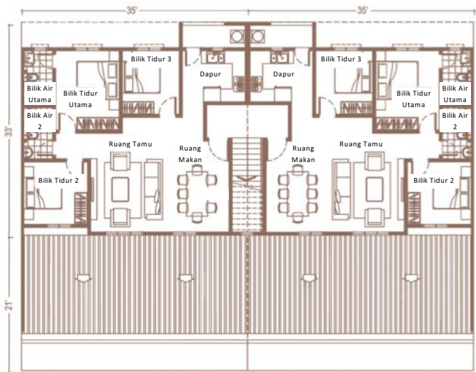
Tingkat Atas
