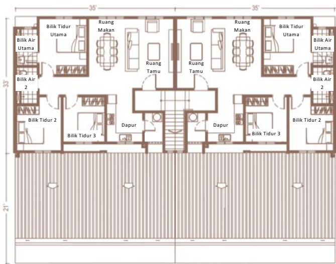
Tingkat Atas
