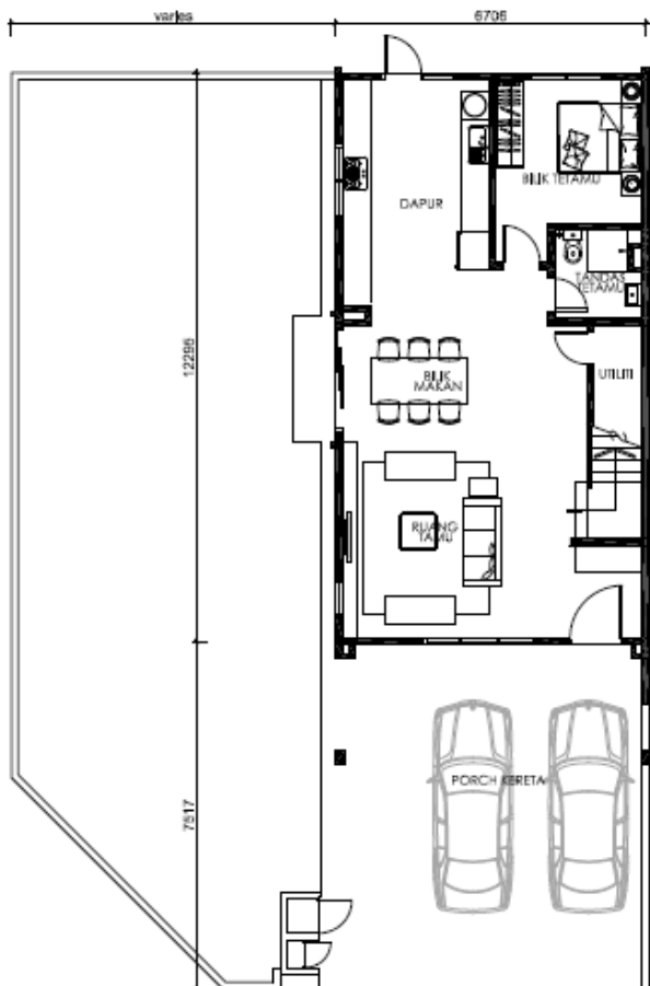
Tingkat Bawah
