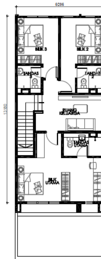
Tingkat Atas
