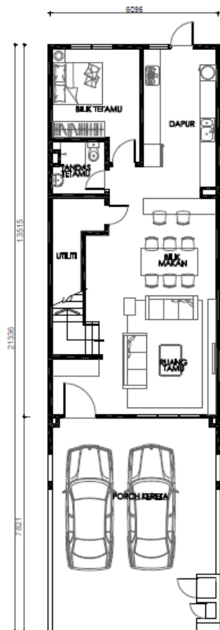
Tingkat Bawah
