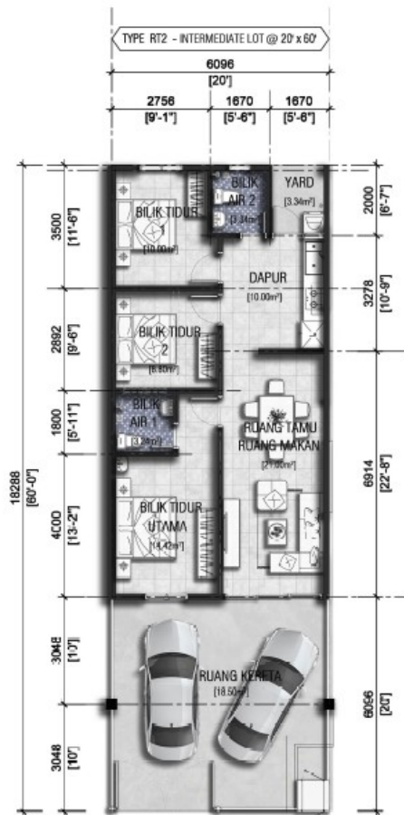
PELAN LANTAI - LOT TENGAH
