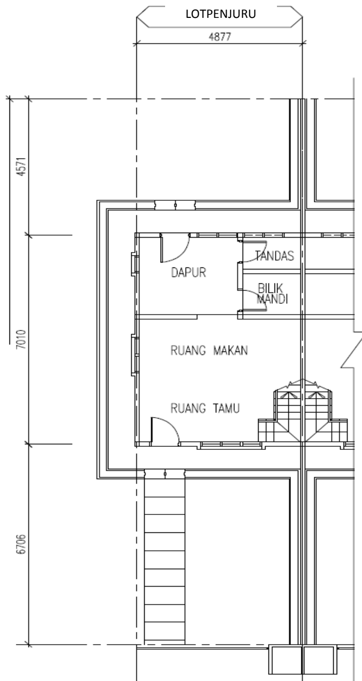
PTD 92920, PTD 92930 & PTD 92939 PELAN TINGKAT BAWAH RUMAH TERES KOMUNITI 2 TINGKAT JENIS A
