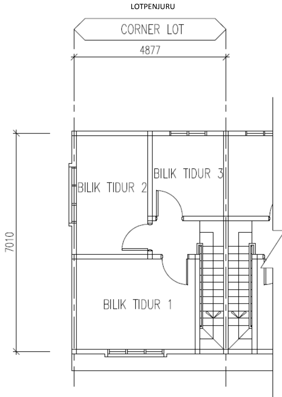
PTD 92920, PTD 92930 & PTD 92939 PELAN TINGKAT SATU RUMAH TERES KOMUNITI 2 TINGKAT JENIS A
