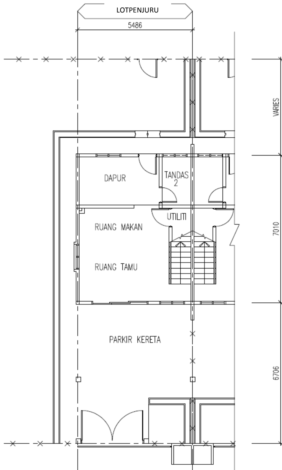
PTD 92966 & PTD 92976 PELAN TINGKAT BAWAH RUMAH TERES KOMUNITI 2 TINGKAT JENIS B
