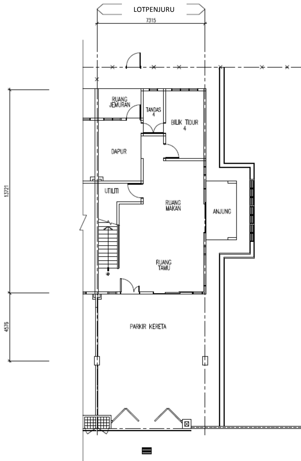
PELAN TINGKAT BAWAH RUMAH TERES 2 TINGKAT
