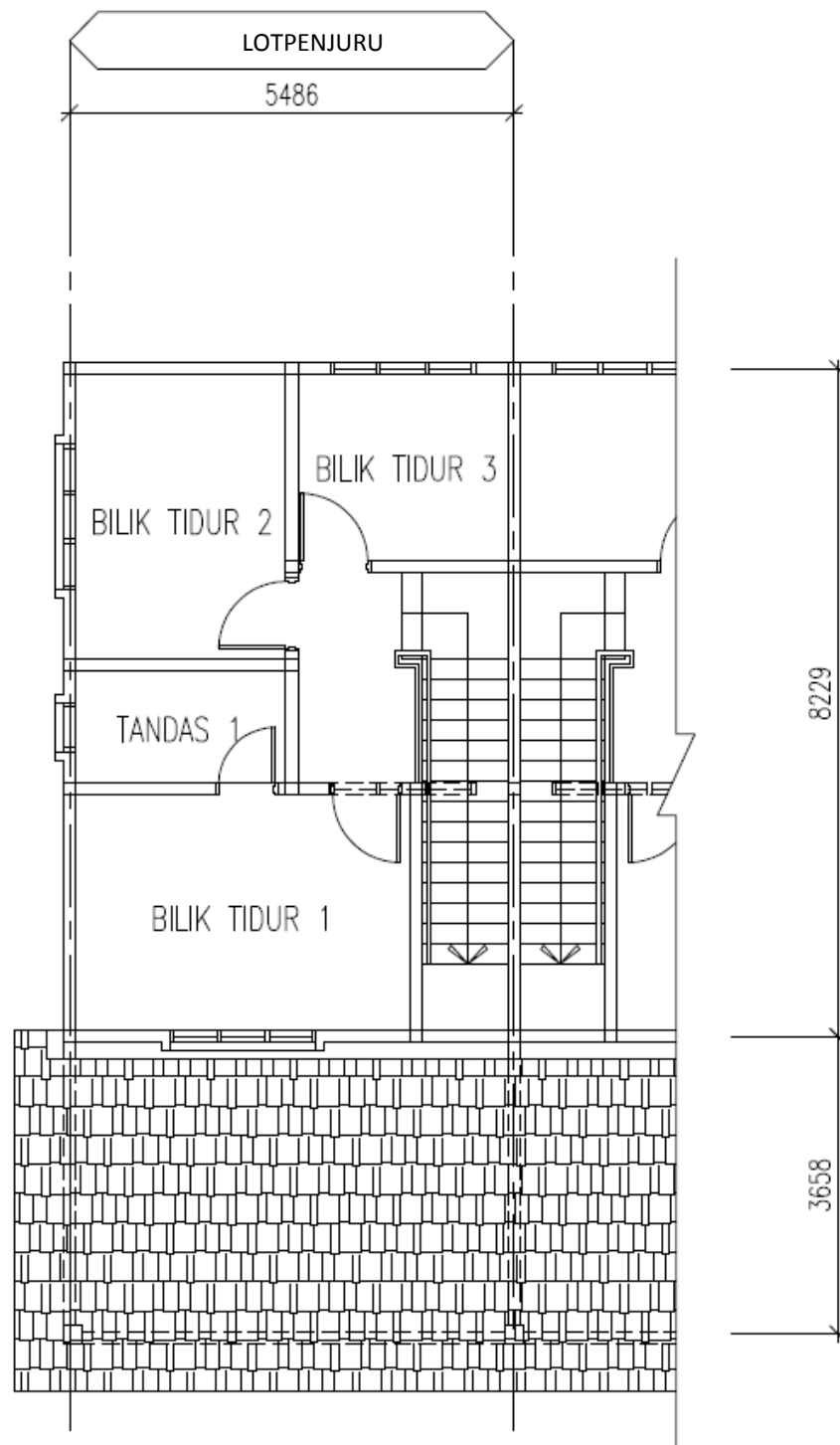
PTD 92966 & PTD 92976 PELAN TINGKAT SATU RUMAH TERES KOMUNITI 2 TINGKAT JENIS B
