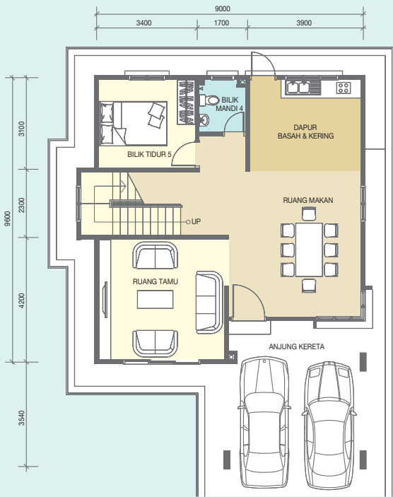
PELAN TINGKAT BAWAH
