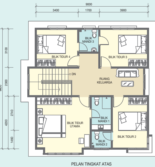
PELAN TINGKAT ATAS
