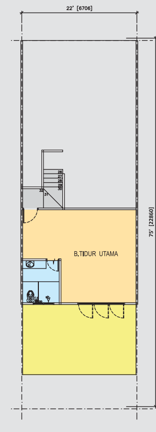
PELAN ARAS DUA (22' x 75')
