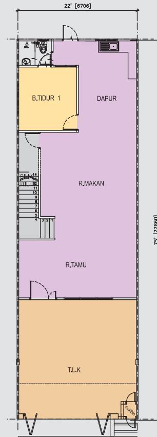
PELAN ARAS TANAH (22' x 75')
