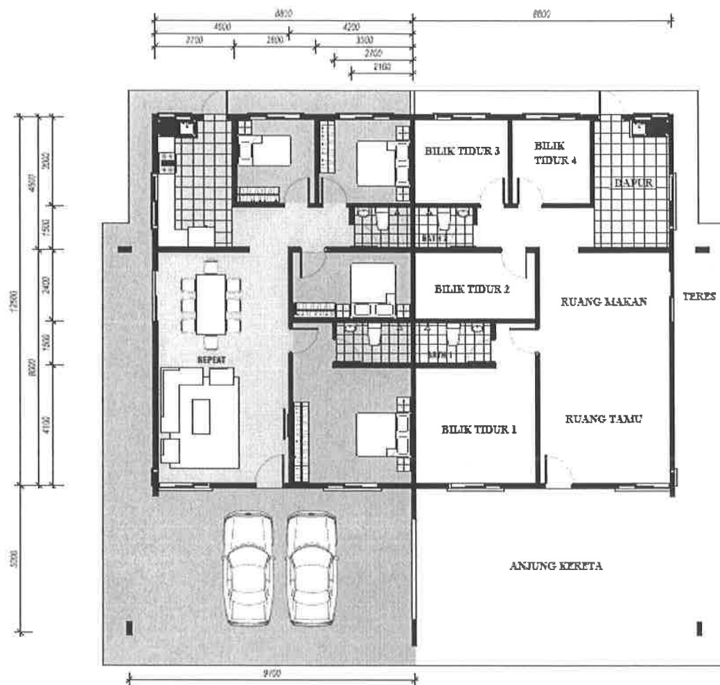
PELAN LANTAI
