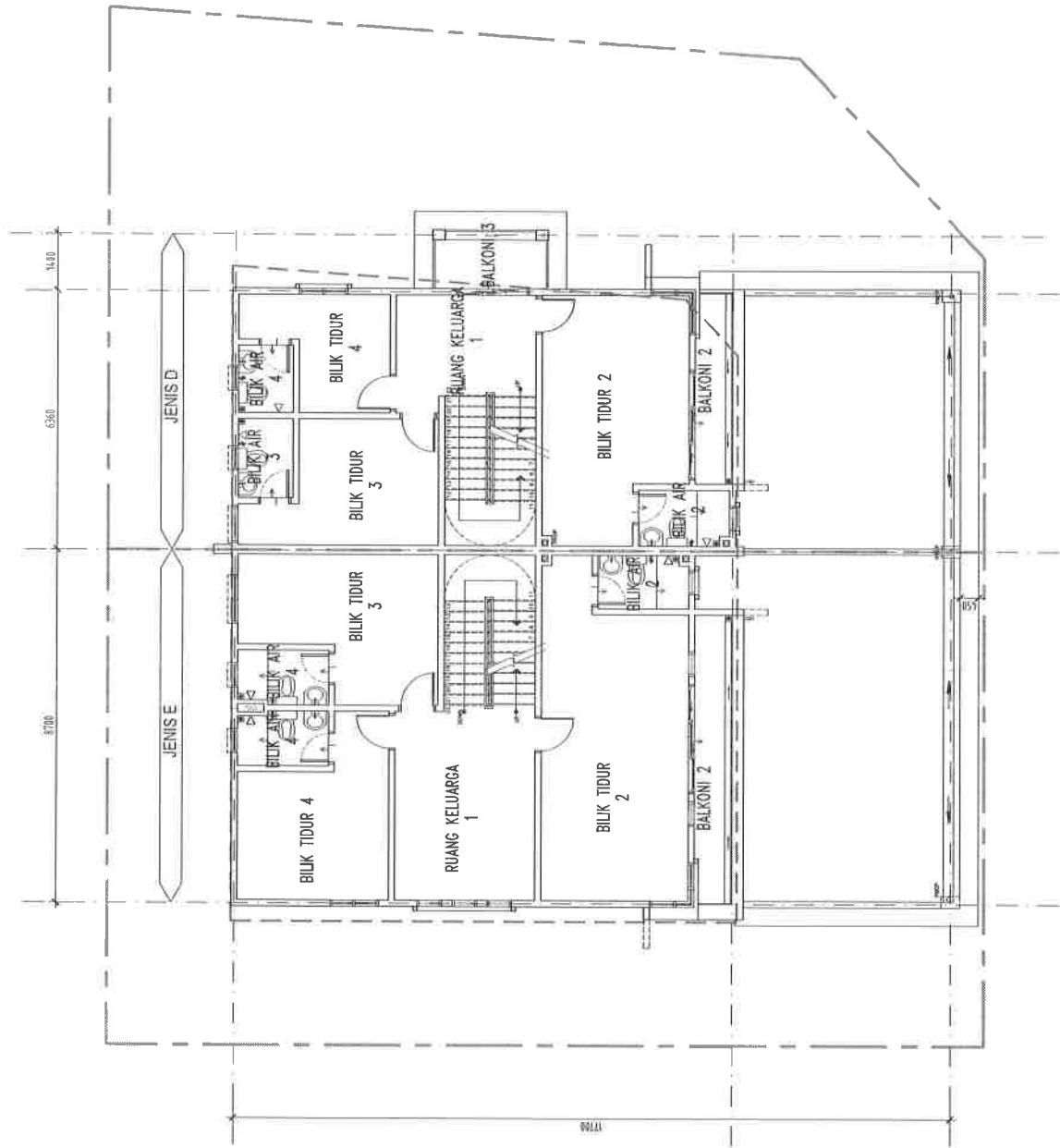
PELAN LANTAI
