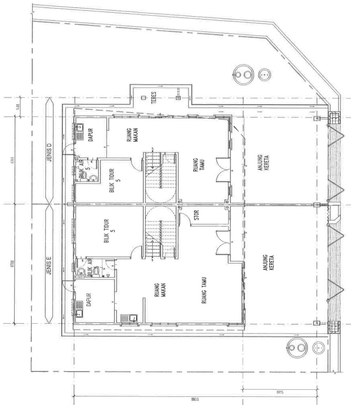
PELAN LANTAI ARAS 1
