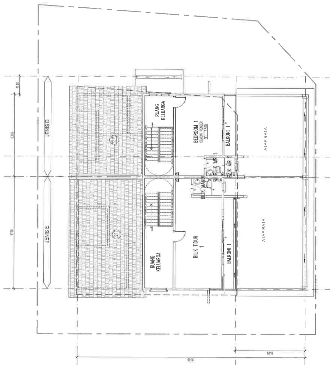
PELAN LANTAI ARAS 2
