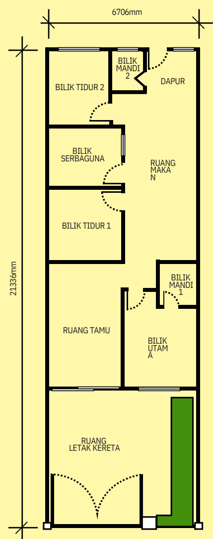
JENIS E : 22' X 70'
