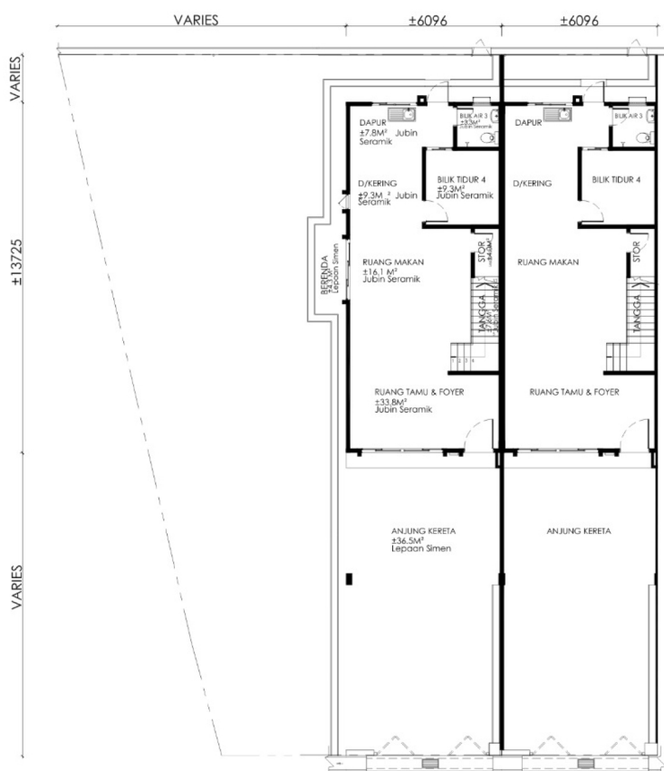
PELAN LANTAI BAWAH
