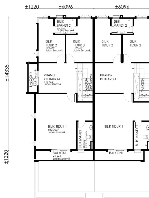
PELAN LANTAI TINGKAT 1
