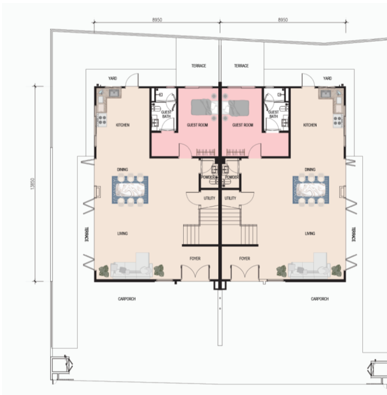
Tingkat Bawah
