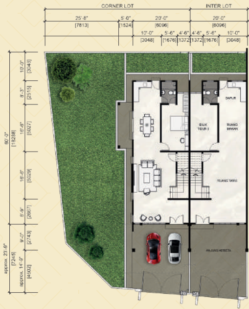
Pelan Tingkat Bawah
