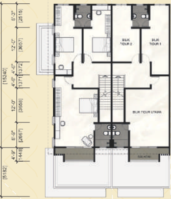
Pelan Tingkat Satu
