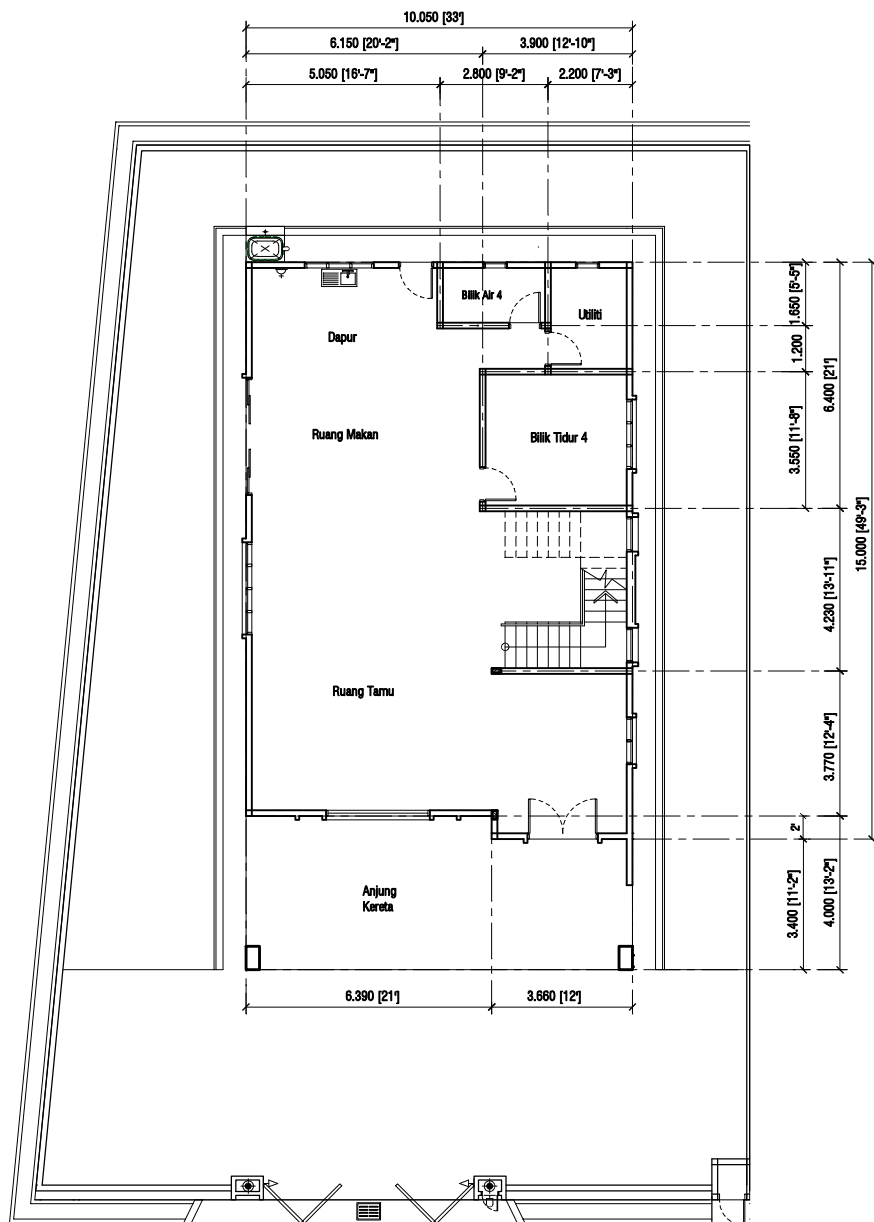
TINGKAT BAWAH
