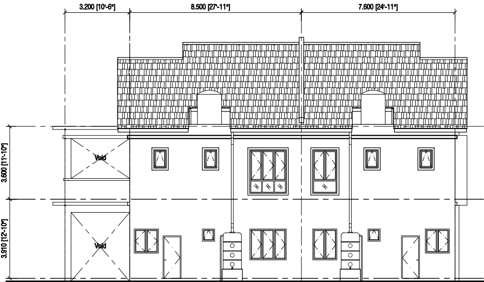
PANDANGAN BELAKANG
