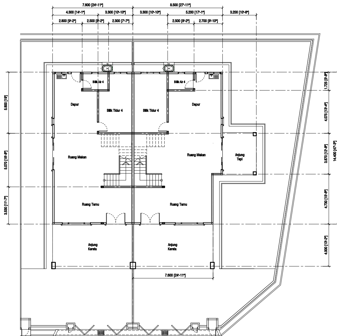
PELAN LANTAI TINGKAT BAWAH
