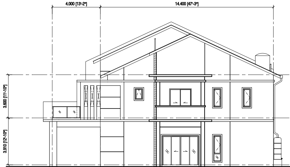
PANDANGAN TEPI
