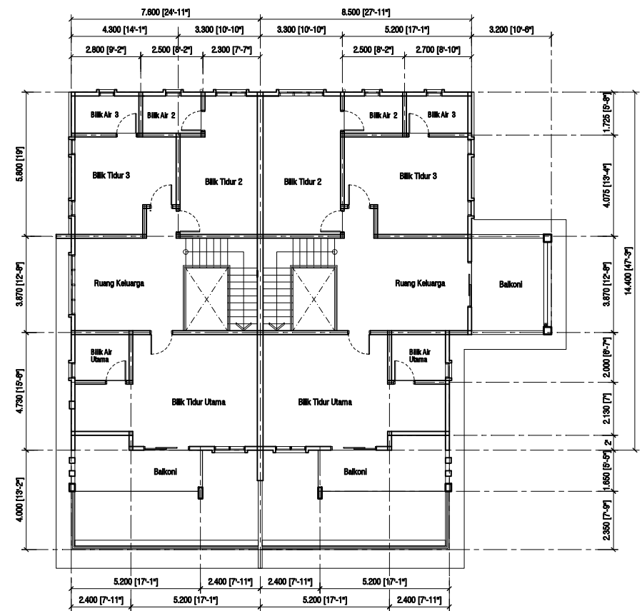
PELAN LANTAI TINGKAT SATU
