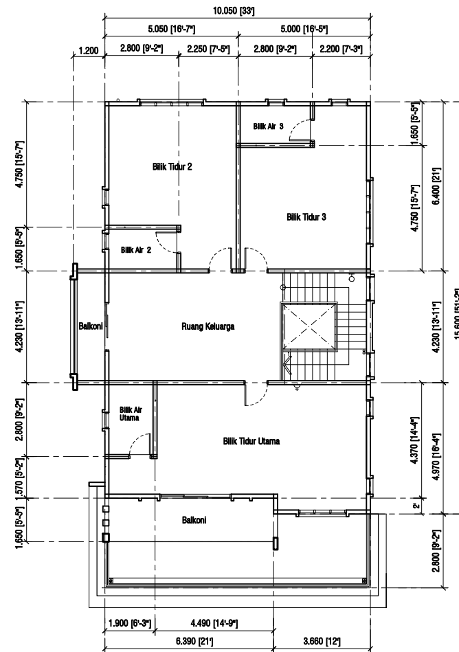
TINGKAT SATU
