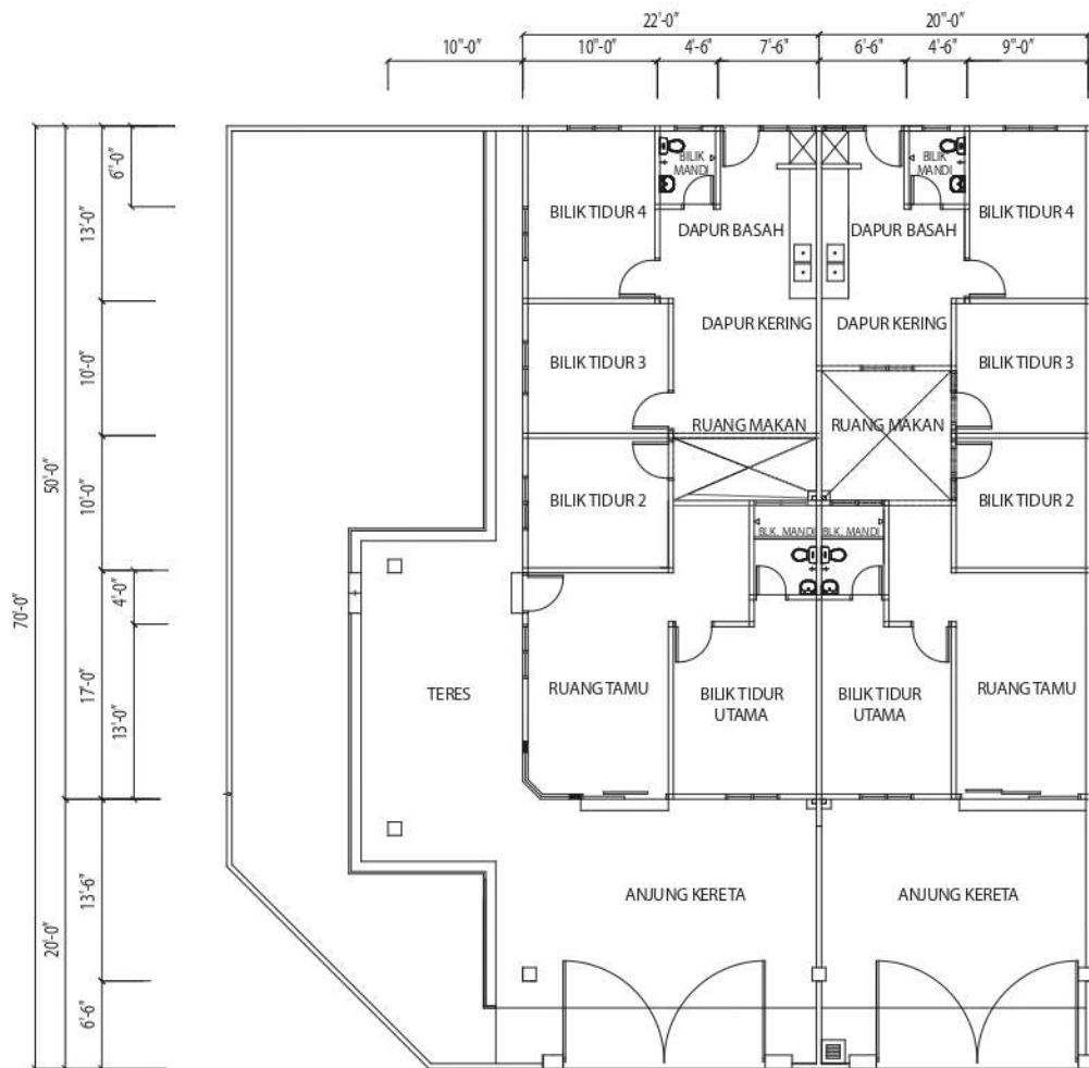
PELAN LANTAI
