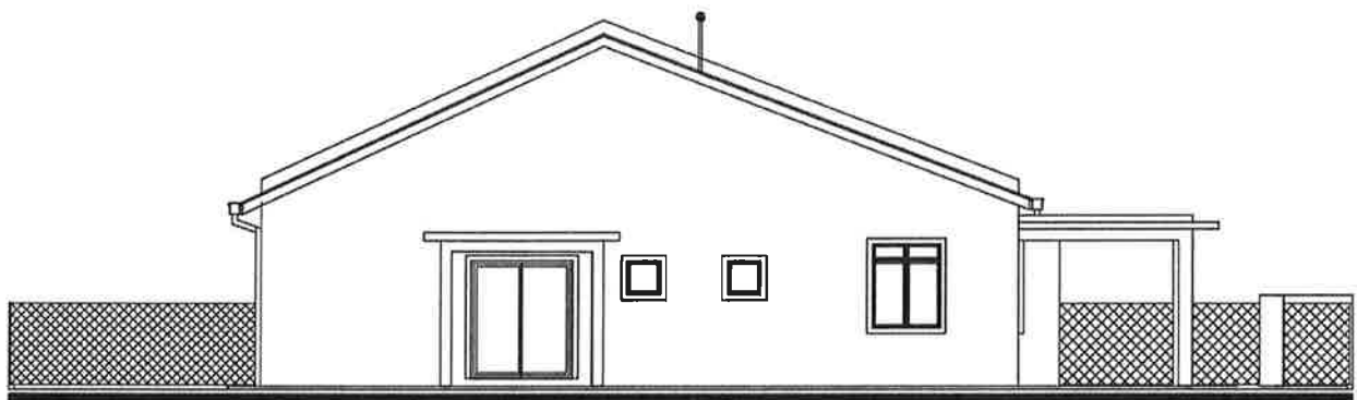
PANDANGAN SISI
