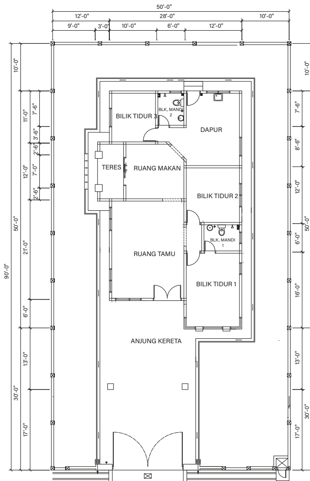
PELAN LANTAI
