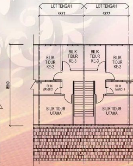
PELAN TINGKAT SATU
