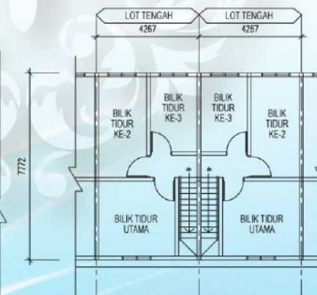
PELAN TINGKAT SATU
