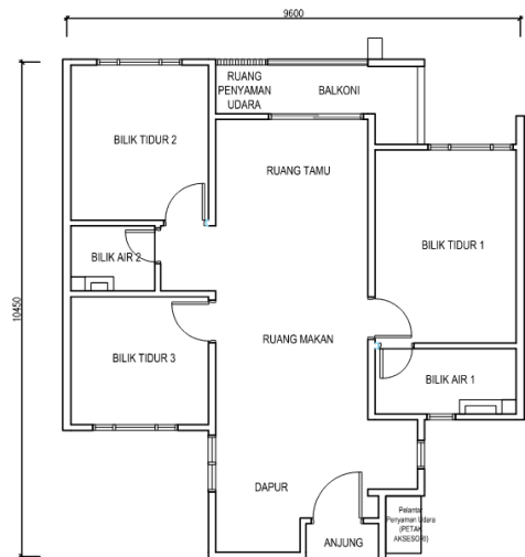
JENIS A (Kanan) 872 KP 3 BILIK TIDUR, 2 BILIK MANDI
