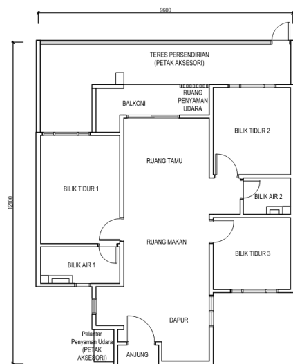
JENIS Aa (Kiri) 872 KP 3 BILIK TIDUR, 2 BILIK MANDI
