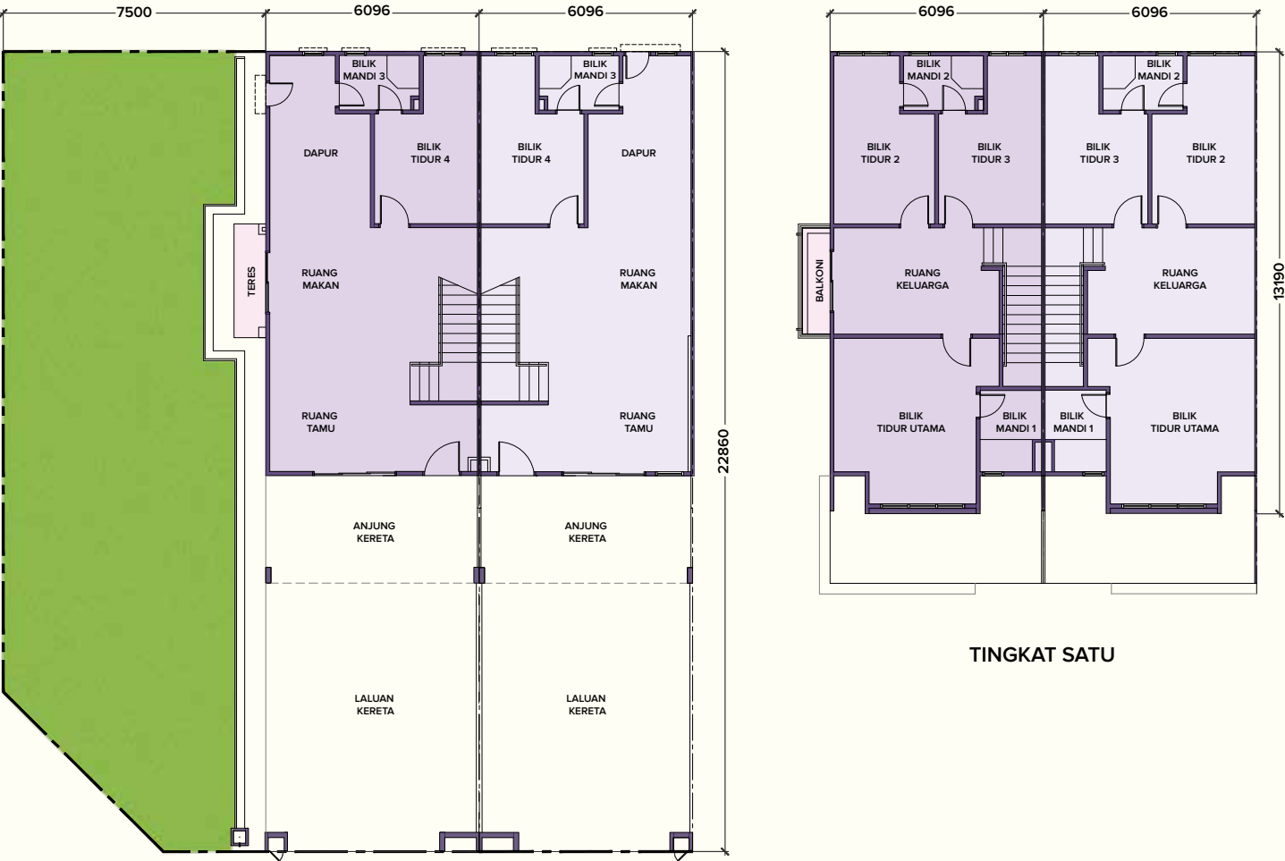
TINGKAT BAWAH
