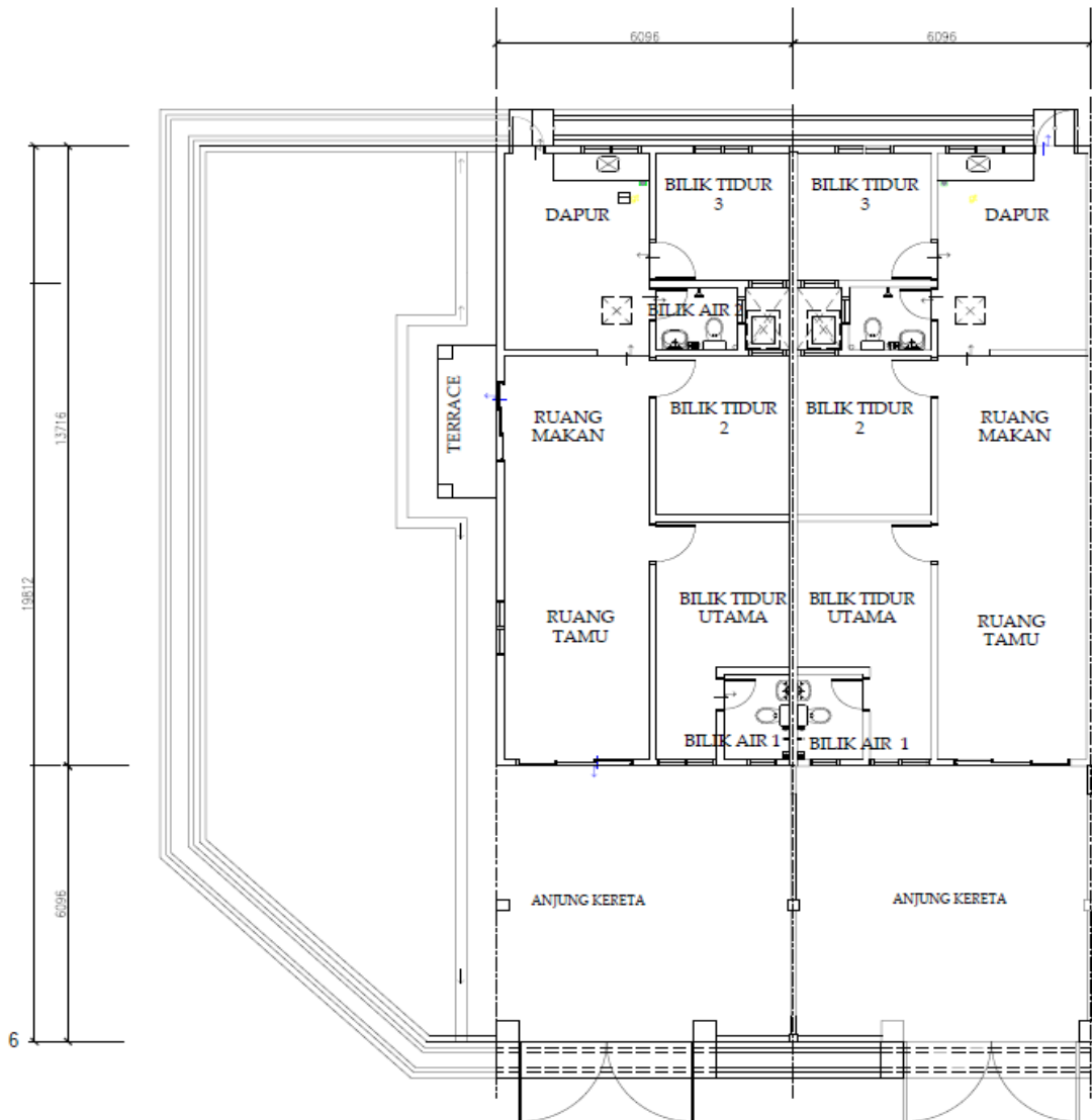
PELAN LANTAI - TYPE A
