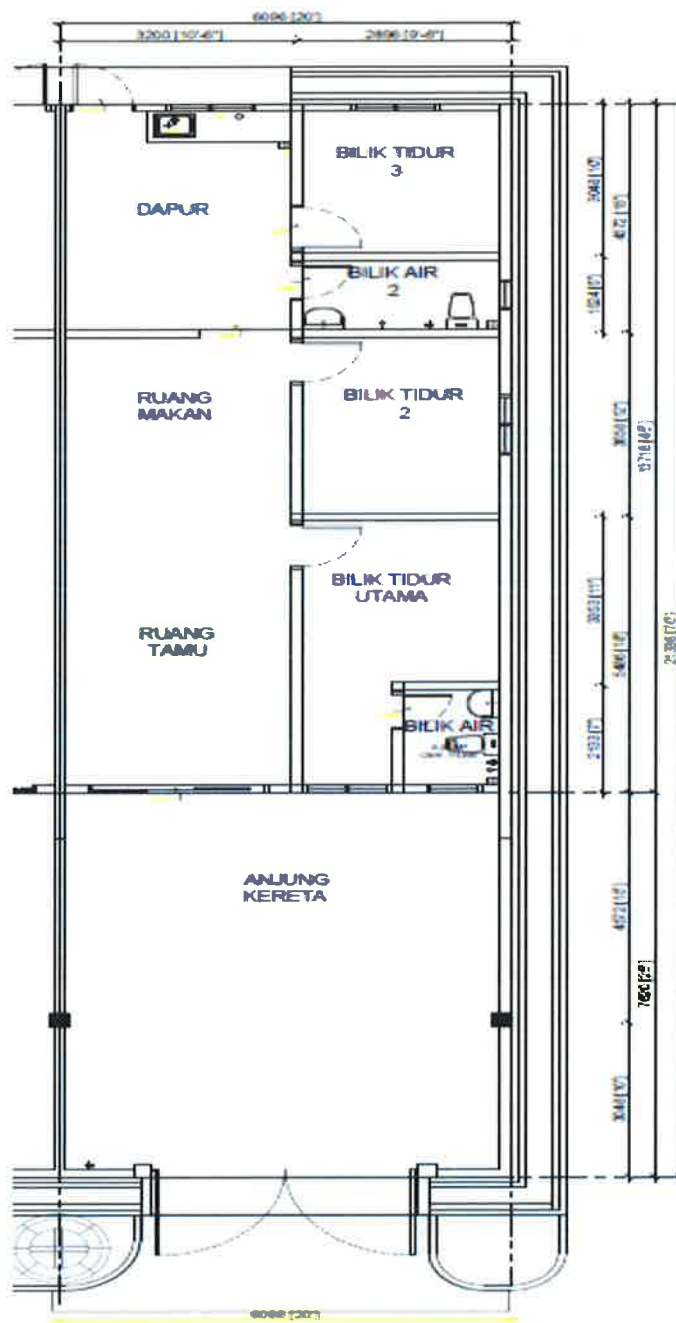
PELAN LANTAI -TYPE A
