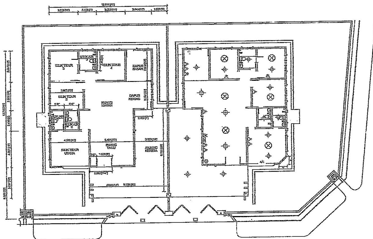
PELAN LANTAI JENIS A
