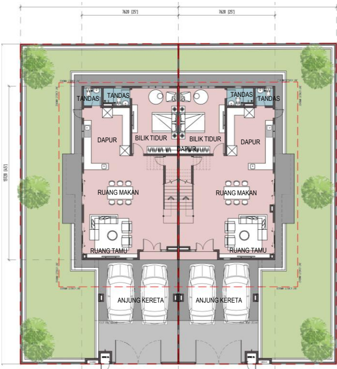
PELAN TINGKAT BAWAH
