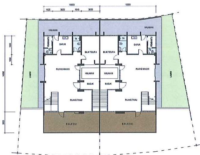
PELAN ARAS LANTAI
