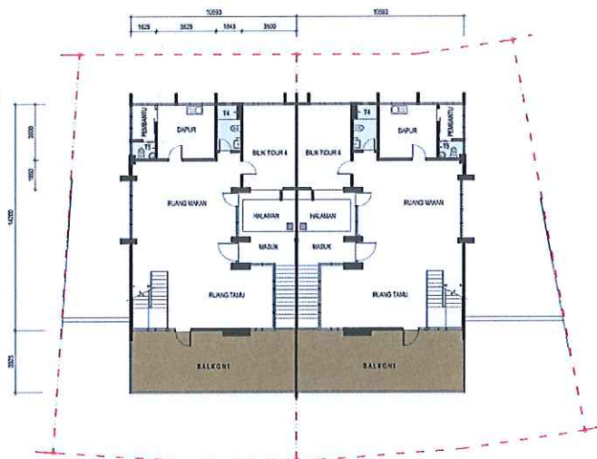
PELAN ARAS LANTAI
