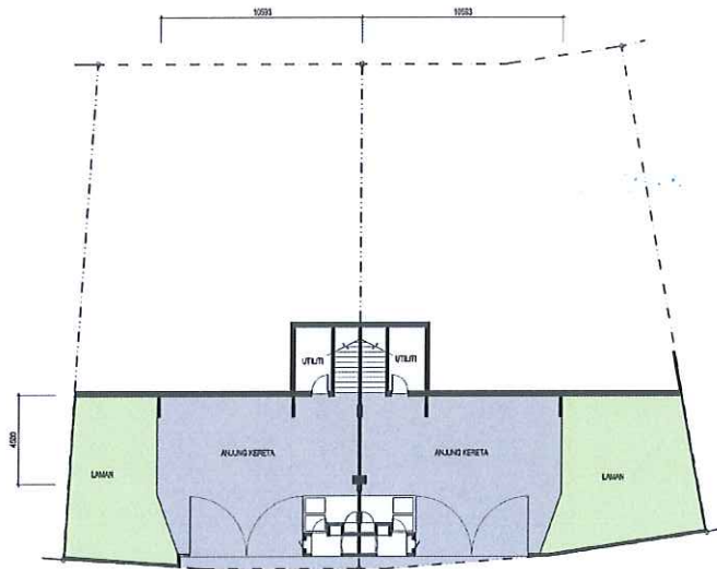
PELAN ARAS ANJUNG KERETA
