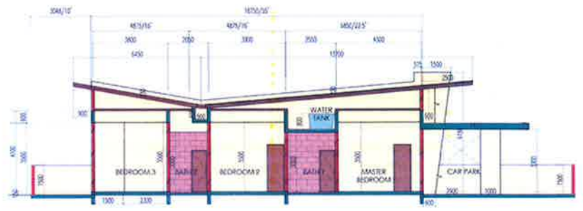
PANDANGAN TEPI
