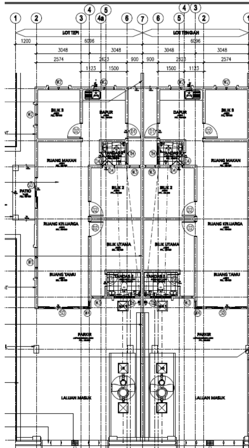
PELAN LANTAI. SCALE : 1:100
