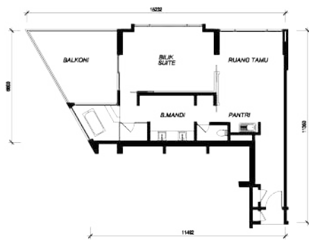
JENIS SS 2 KELUASAN BINAAN 1065 K.P.
