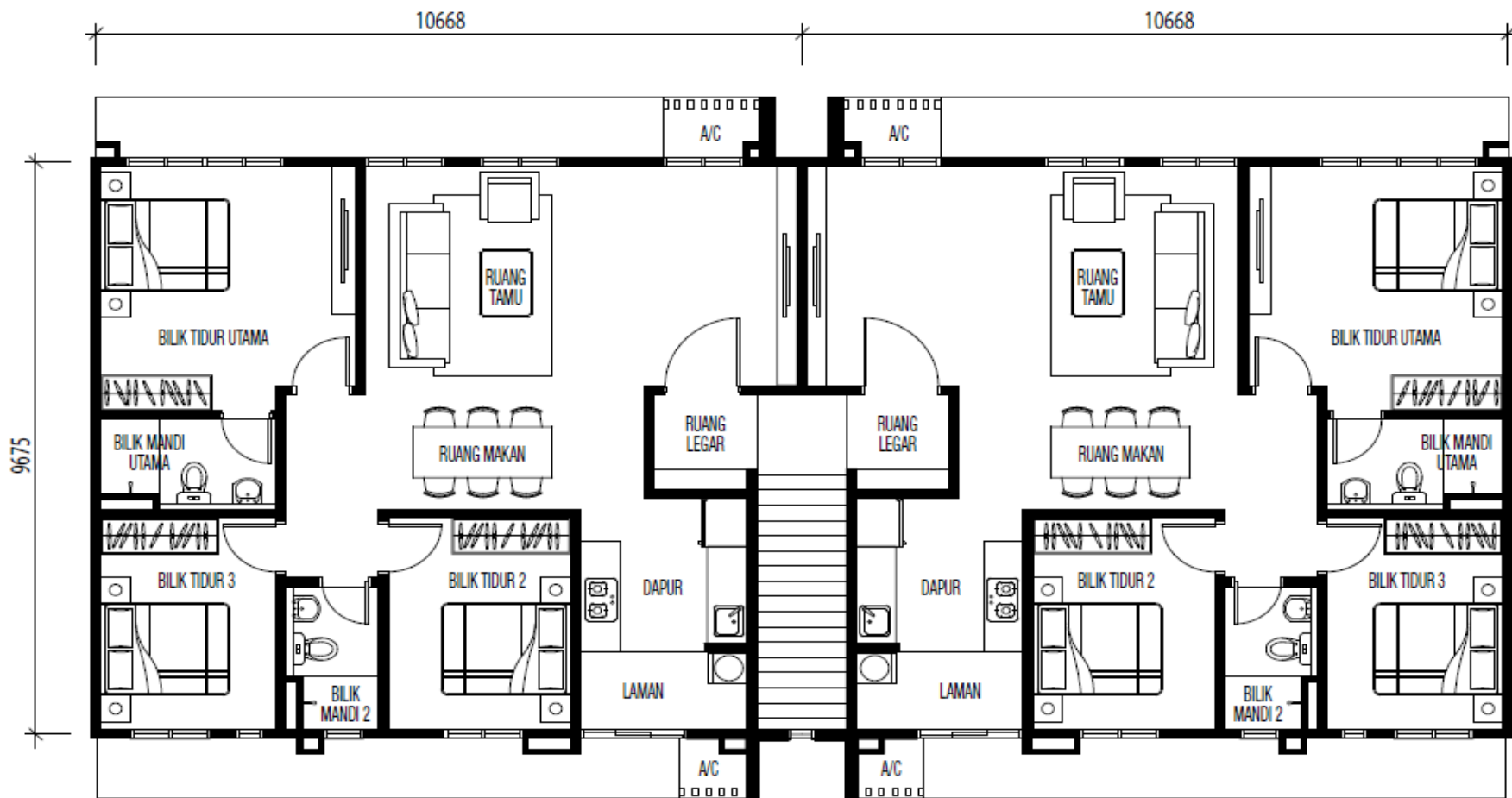
TINGKAT ATAS
