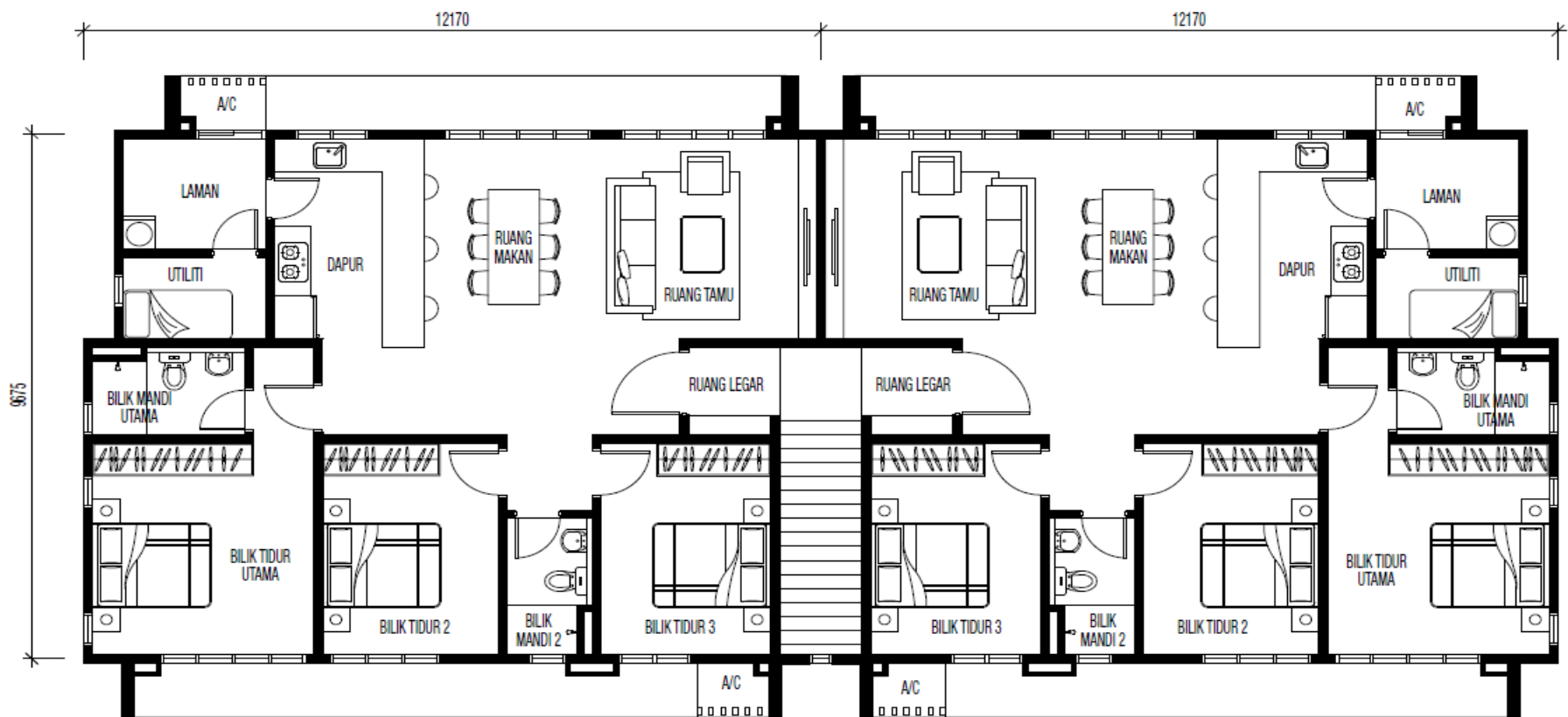
TINGKAT ATAS
