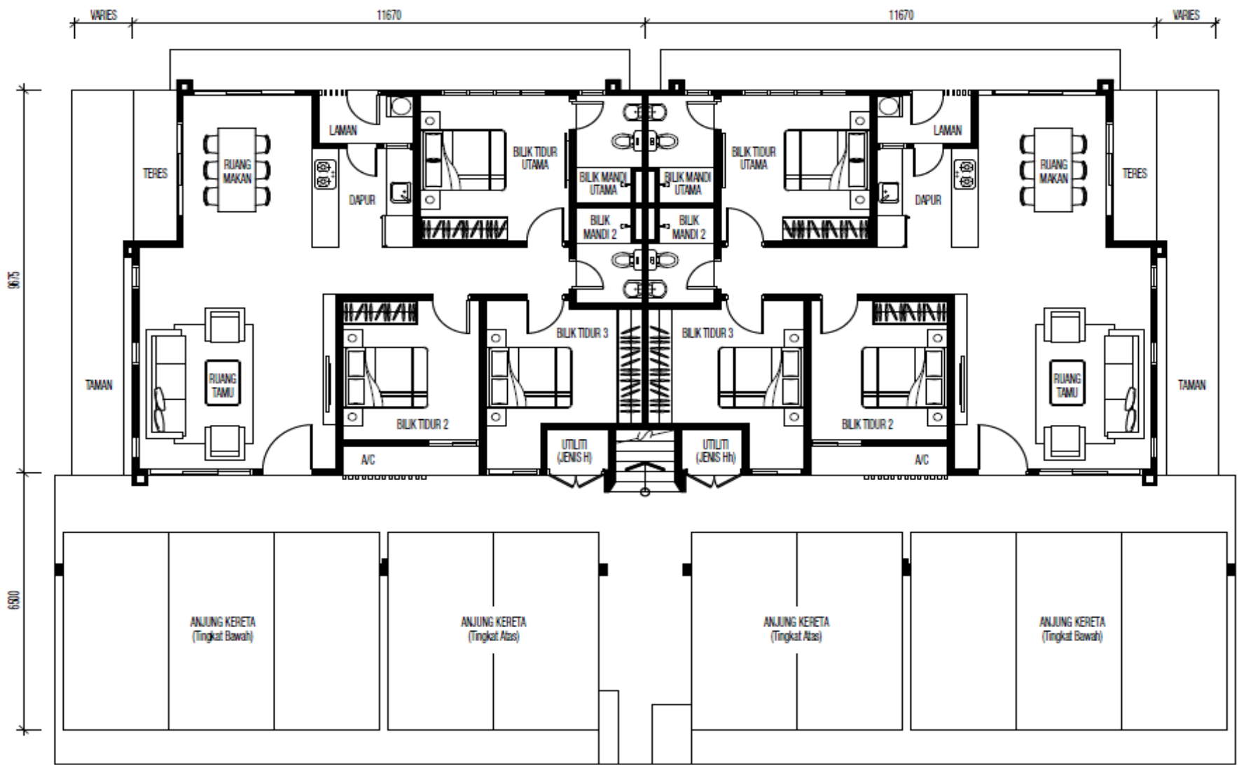
TINGKAT BAWAH
