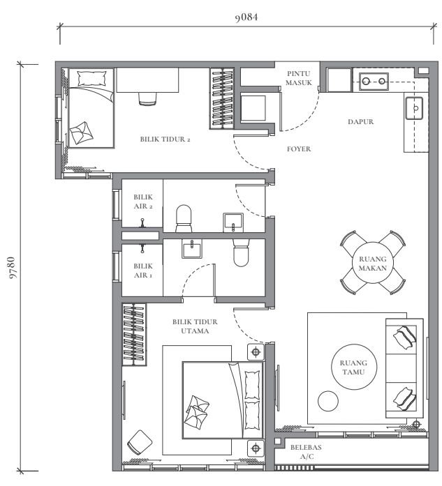
JENIS A1 /A2 812 kps 2 Bilik Tidur | 2 Bilik Air
