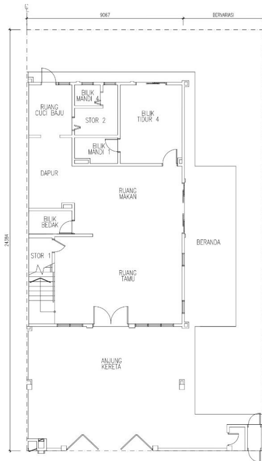
ARAS BAWAH
